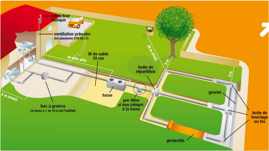
Installation avec tranchées d'épandage
